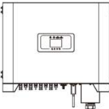
Figura 1.1 Vista frontal
